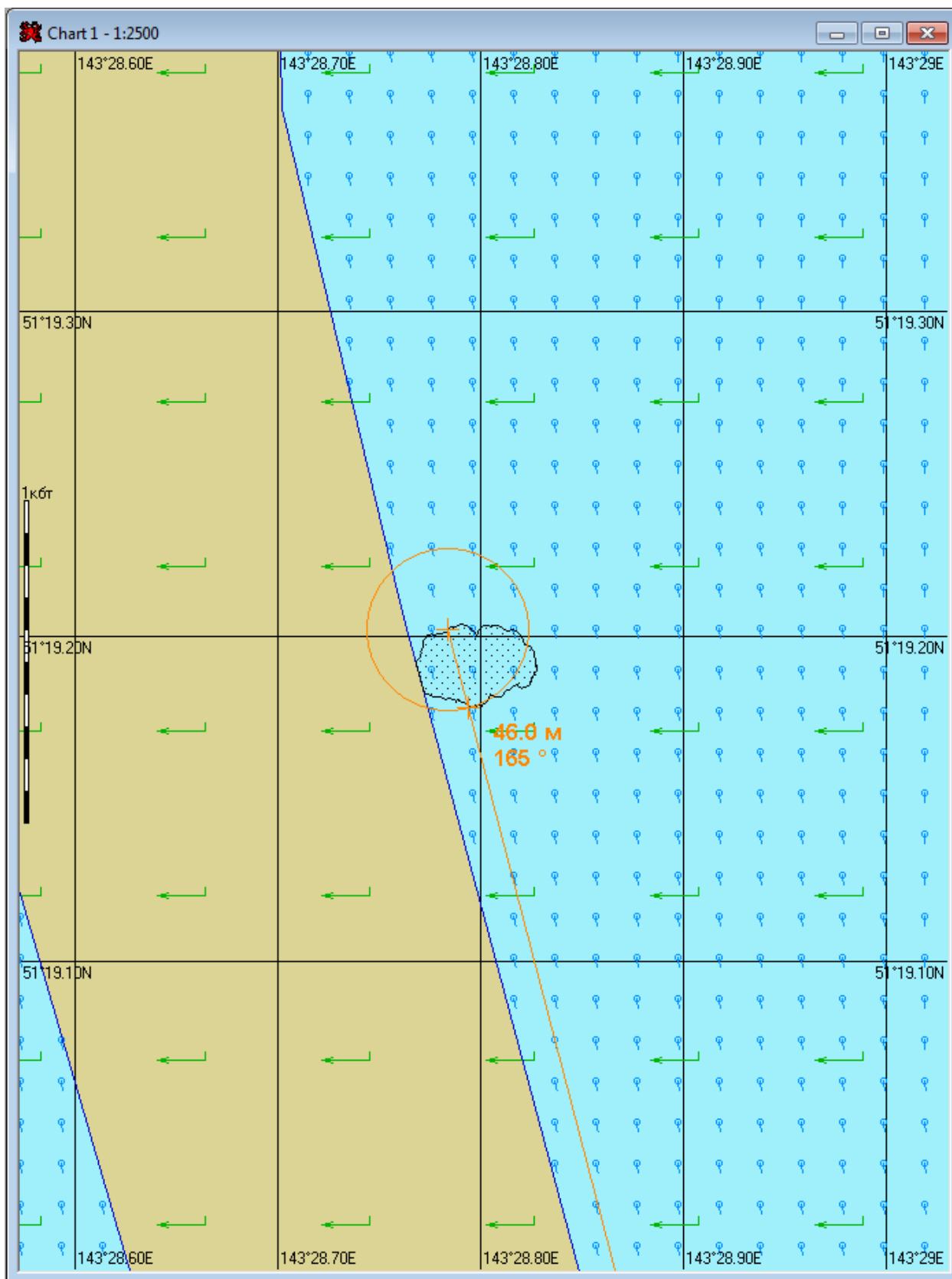
Рис. 2.6. Карта ЧС(Н) на момент достижения нефтяным пятном берега (26ч 15мин) при восточном ветре и скорости ветра 5 м/с.
