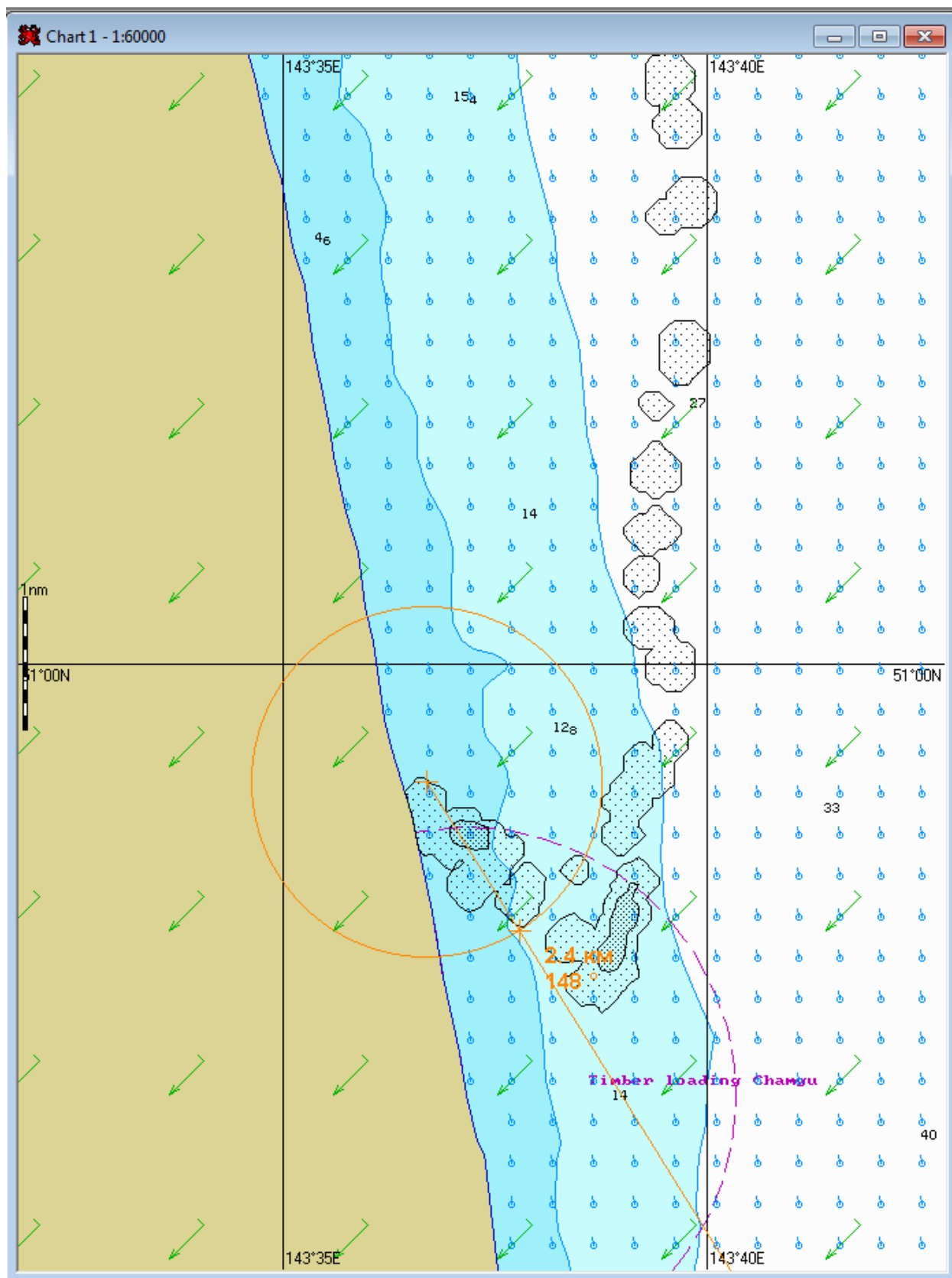
Рис. 2.11. Карта ЧС(Н) на момент достижения нефтяным пятном берега (53ч 20мин) при северо-восточном ветре и скорости ветра 5 м/с.
