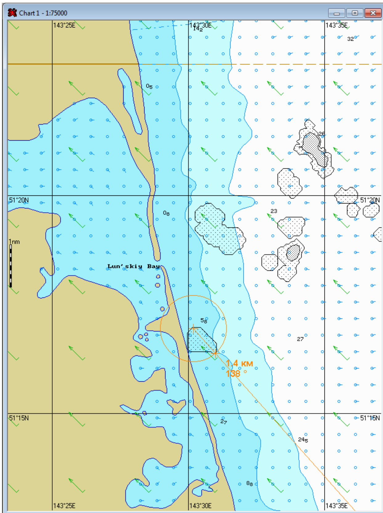
Рис. 2.9. Карта ЧС(Н) на момент достижения нефтяным пятном берега (77ч 45мин) при юго-восточном ветре и скорости ветра 5 м/с.
