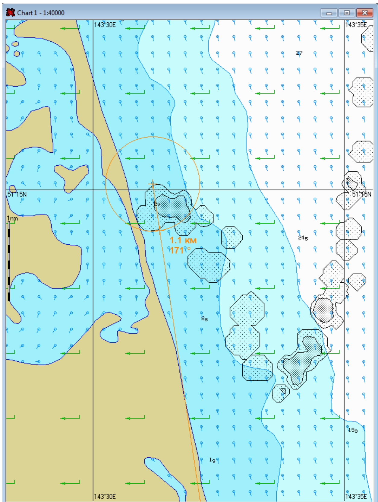
Рис. 2.10. Карта ЧС(Н) на момент достижения нефтяным пятном берега (48ч 30мин) при восточном ветре и скорости ветра 5 м/с.
